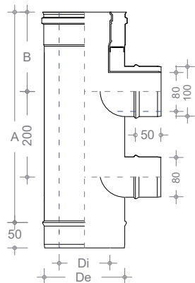
Art. C.90.SV - Raccordo a "T" 90° sdoppiato vert. 90° tee vertically split
