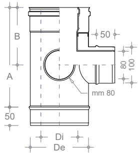
Art. C.90.SOD - Raccordo a "T" 90° sdoppiato orizz. a dx 90° tee horizontally split on the right
